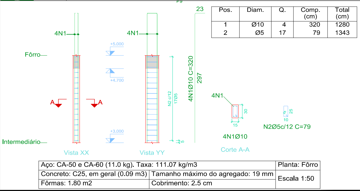
06 Esc FÔRRO 1:50 P9
