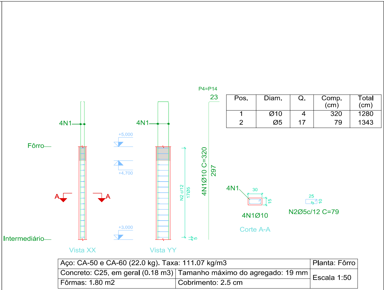
02 Esc FÔRRO 1:50 P4, P14
