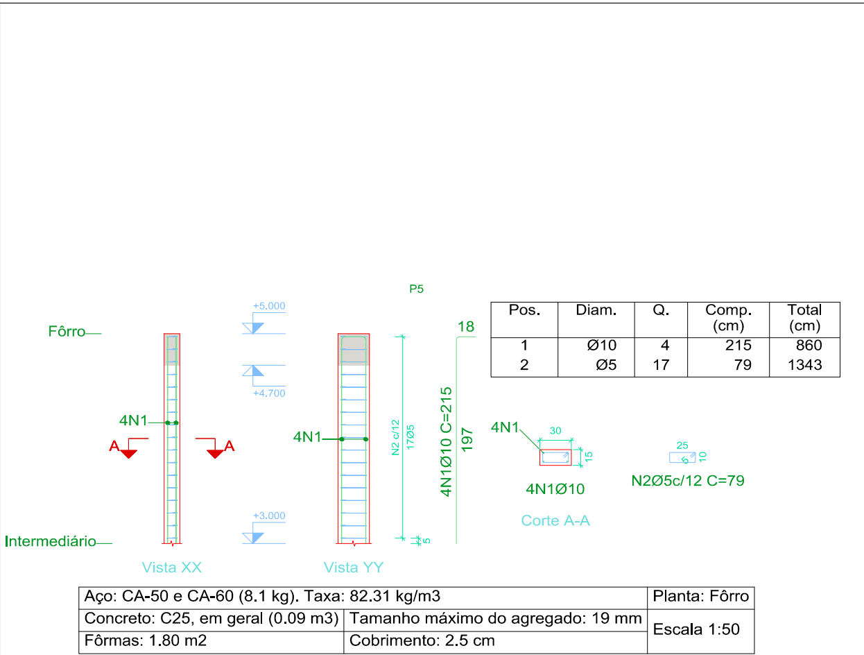
03 Esc FÔRRO 1:50 P5
