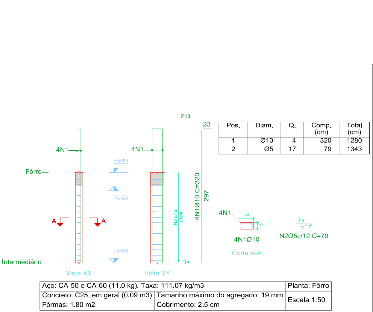
09 Esc FÔRRO 1:50 P13
