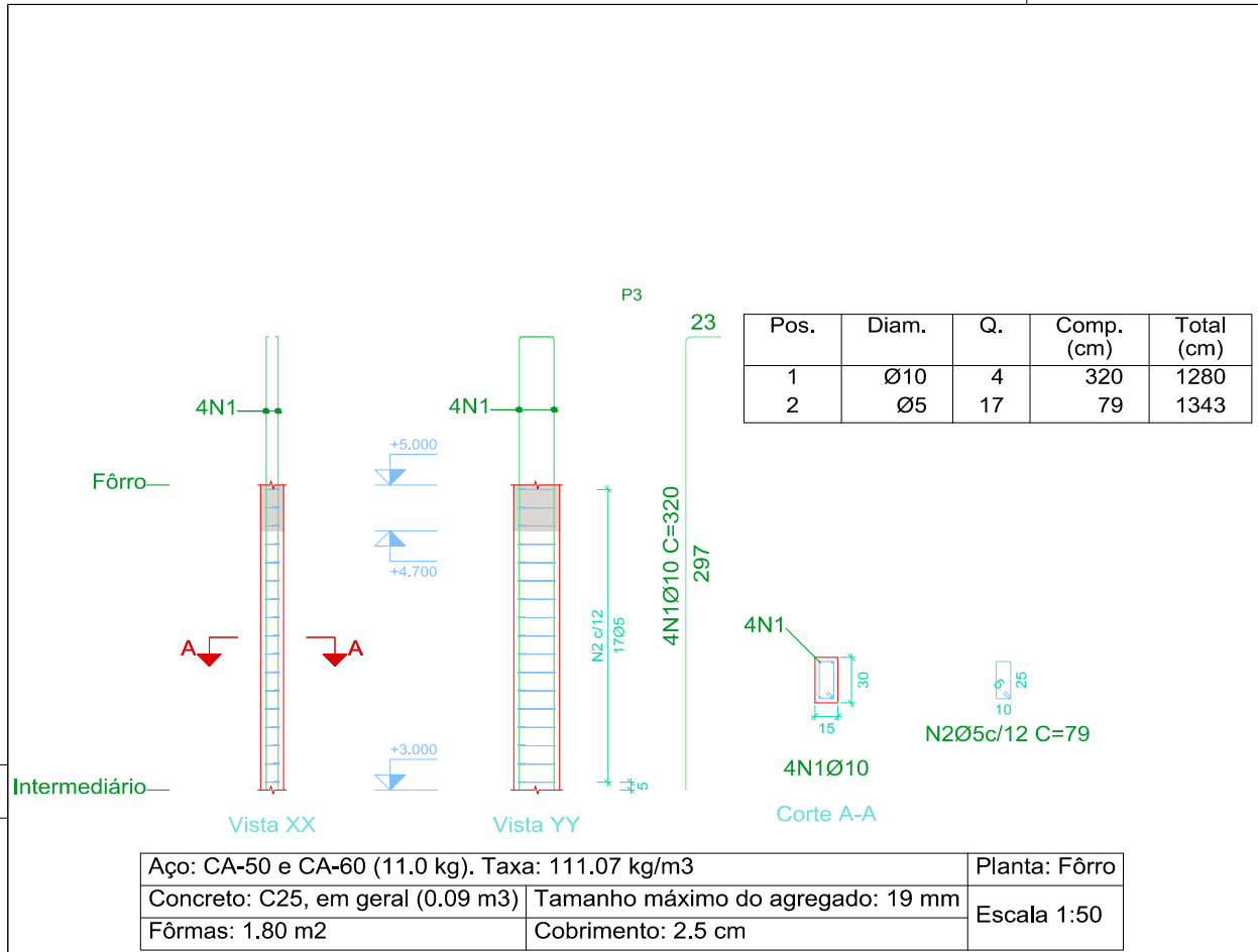
01 Esc FÔRRO 1:50 P3
