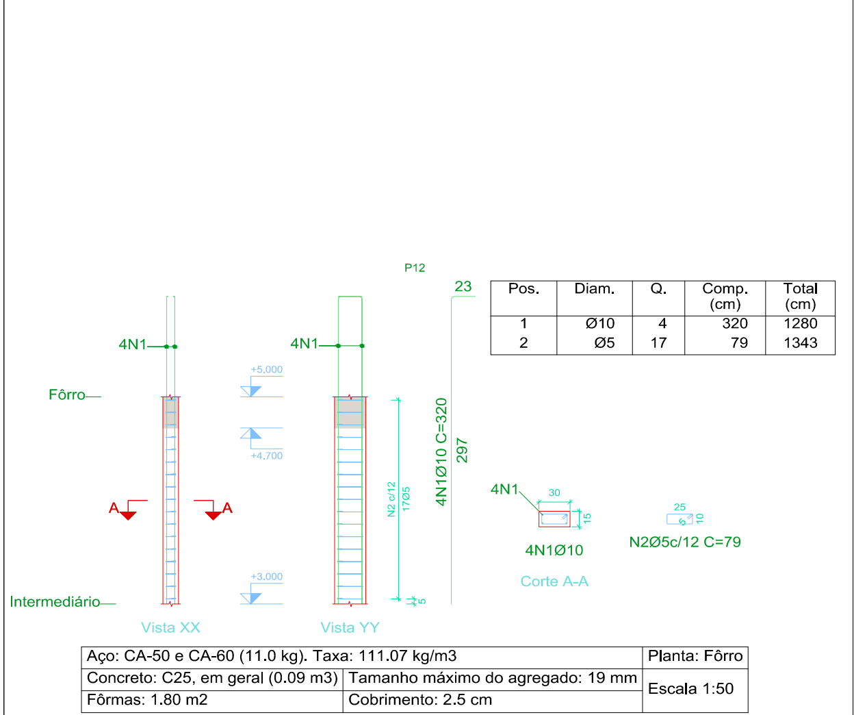
08 Esc FÔRRO 1:50 P12
