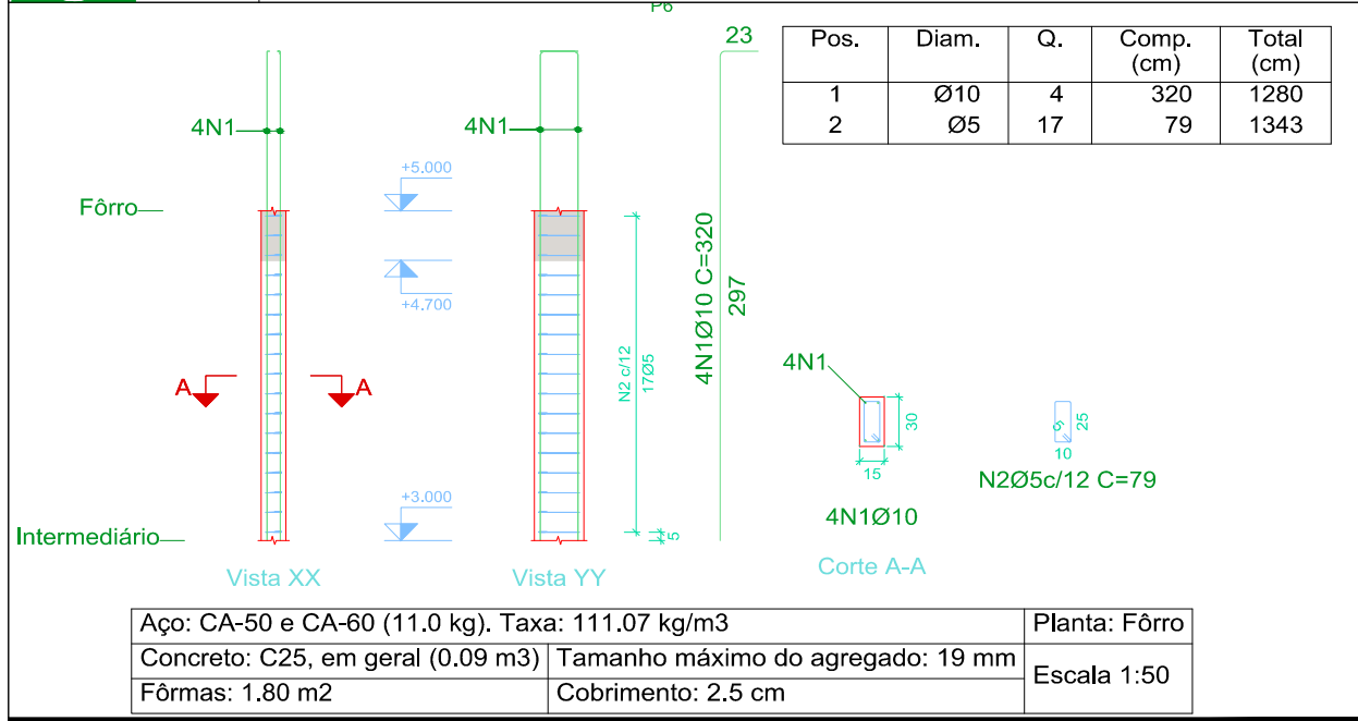
04 Esc FÔRRO 1:50 P6
