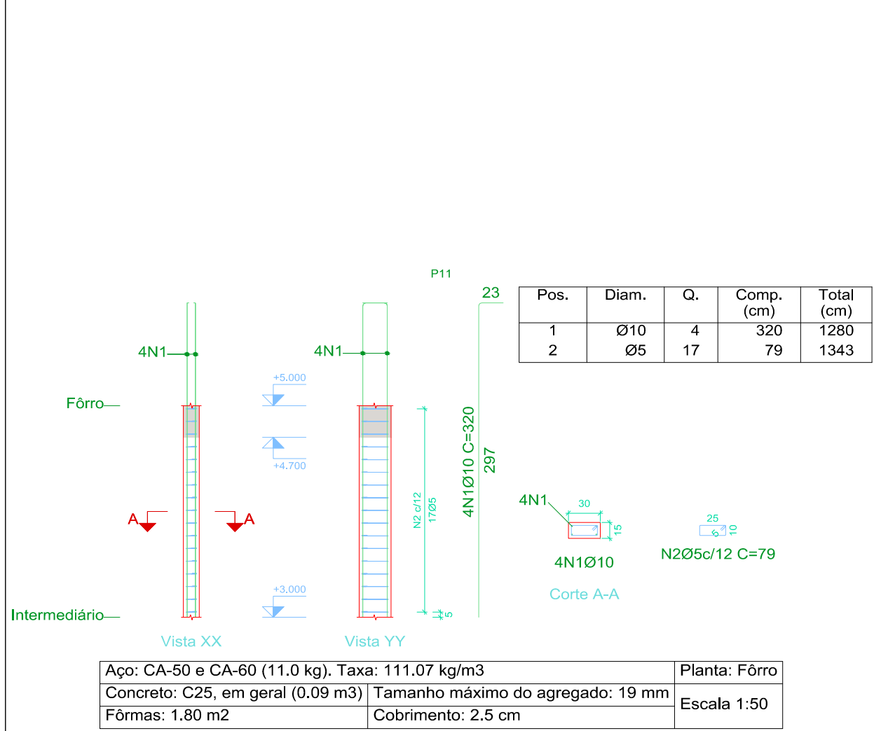
07 Esc FÔRRO 1:50 P11
